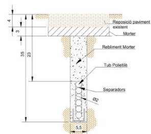
SECCIÓ TRANSVERSAL ST8
