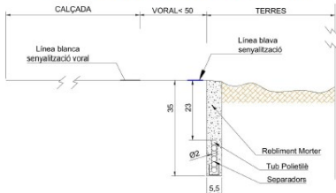
SECCIÓ TRANSVERSAL ST3a
