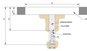
SECCIÓ TRANSVERSAL ST7
