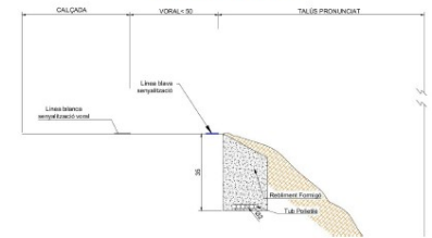
SECCIÓ TRANSVERSAL ST5
