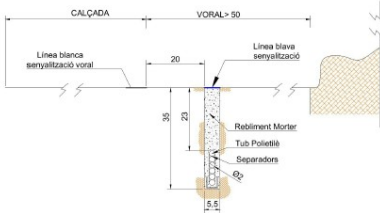
SECCIÓ TRANSVERSAL ST1
