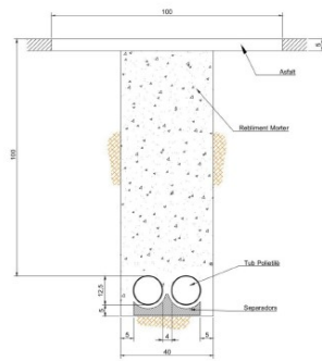
SECCIÓ TRANSVERSAL ST6
