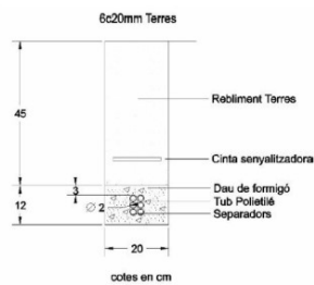
SECCIÓ TRANSVERSAL CC EN TERRES
