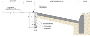
SECCIÓ TRANSVERSAL ST2a
