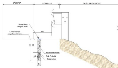
SECCIÓ TRANSVERSAL ST4
