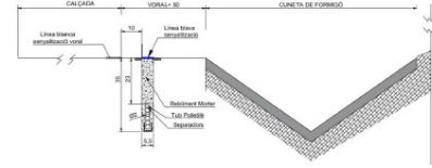
SECCIÓ TRANSVERSAL ST2b
